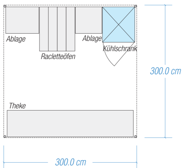
Grundriss mit möglicher Infrastruktur
